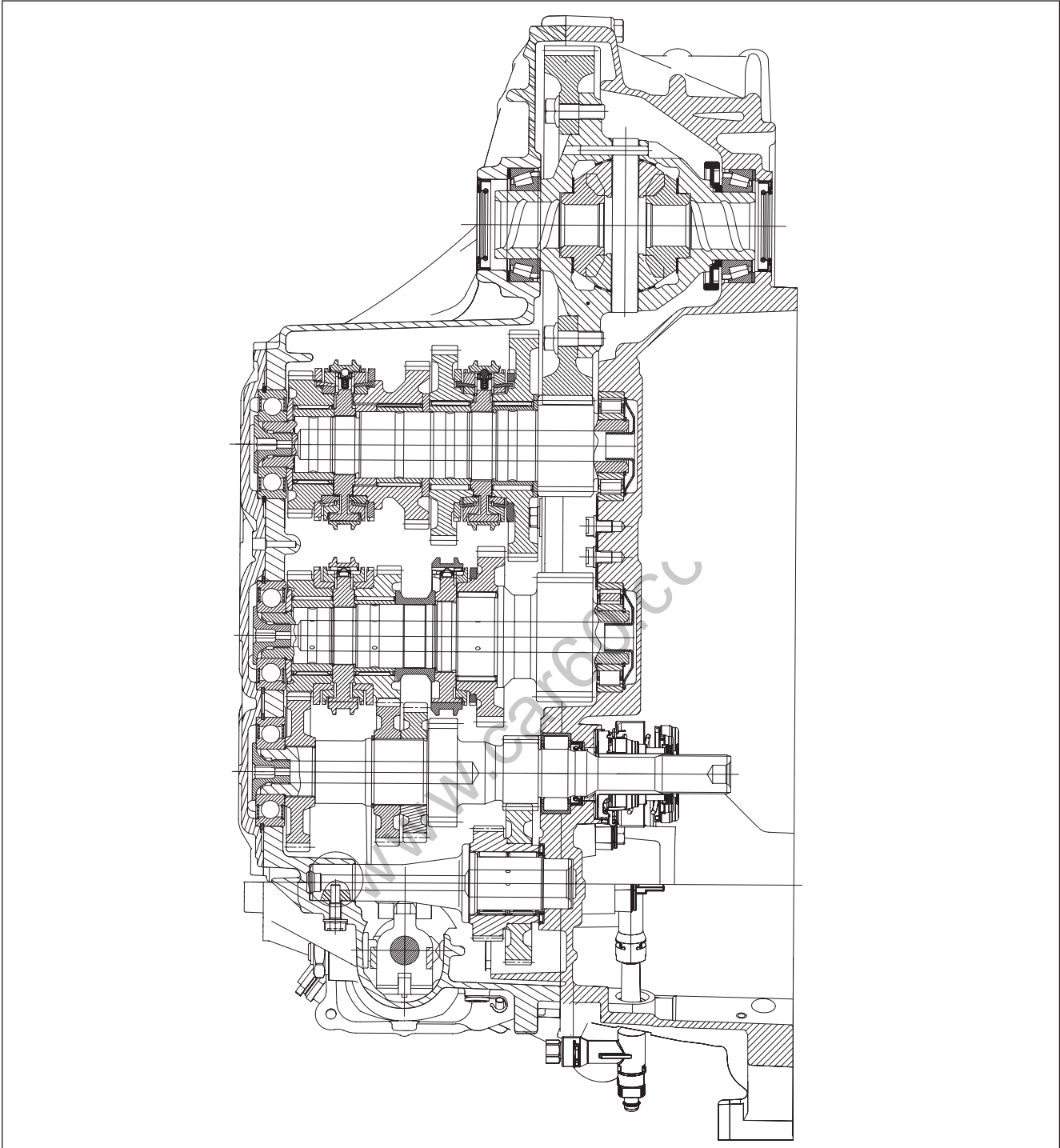
截面图
